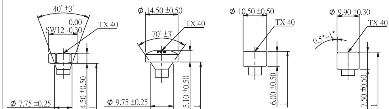
Sechskantkopf mit Torx
