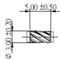
Schaftfräser
