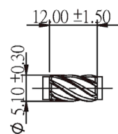
Schaftfräser
