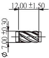
Schaftfräser
