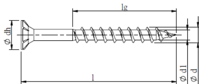
Teilgewinde ohne Bohrspitze
