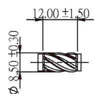
Schaftfräser
