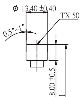
Breiter Zylinderkopf
