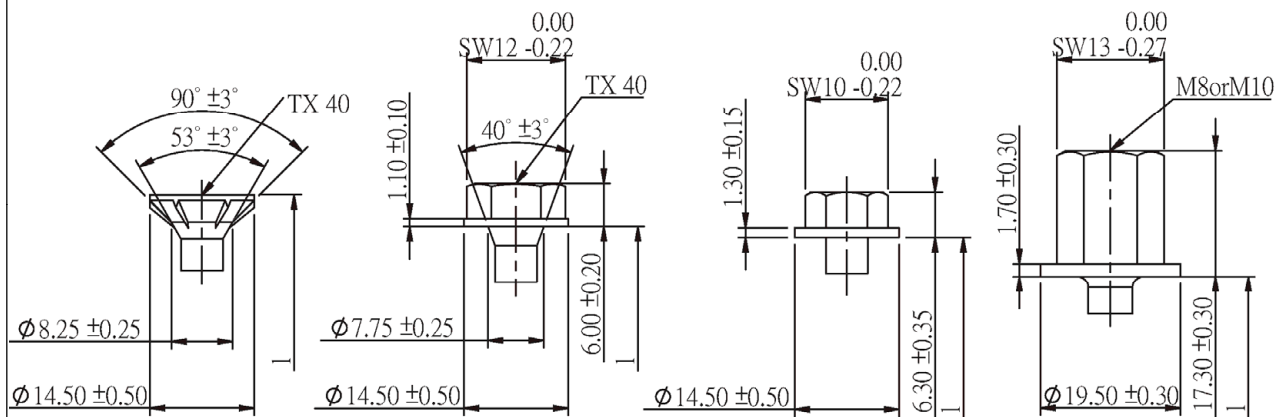
Sechskantkopf mit angepresster Scheibe und Innengewindehülse
