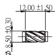
Schaftfräser
