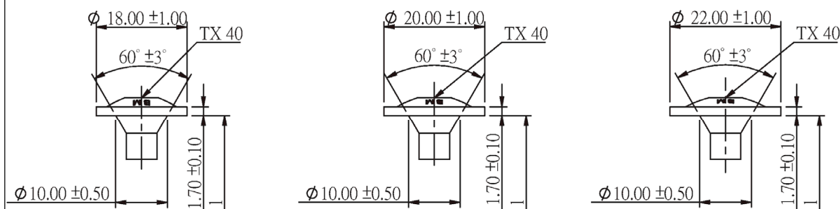
Kleiner Tellerkopf
