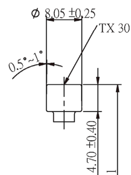
Breiter Zylinderkopf
